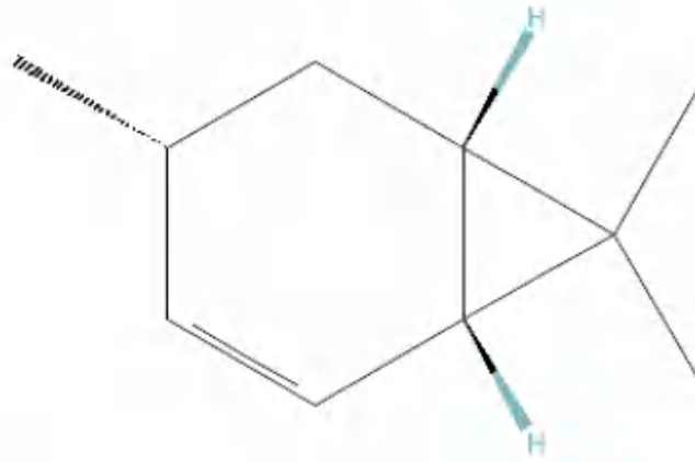
Gambar 4.5 Struktur senyawa (1S,3R,6R)-(-)-4-Carene 2D dalam Teh Baper
