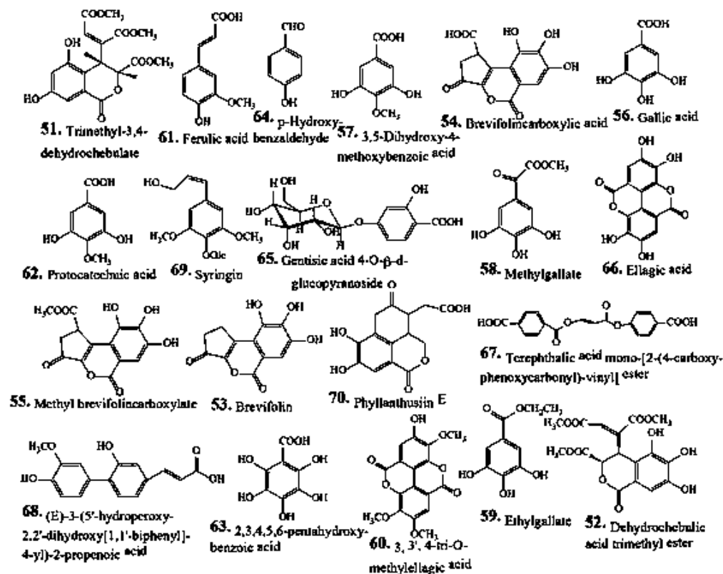
Gambar 3.9 Struktur kimia senyawa fenol dari tanaman meniran (Geethangili & Ding, 2018).
