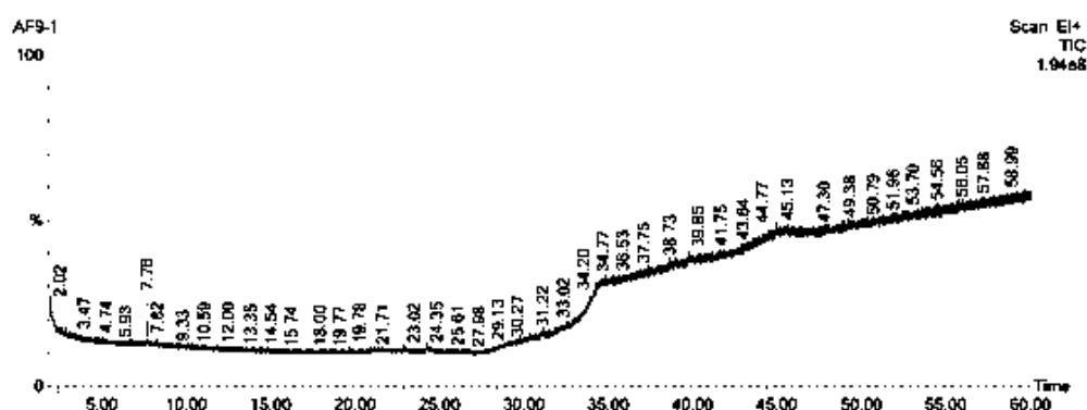
Gambar 4.2 Karakterisasi senyawa dari polyherbal Teh Baper dengan analisis GC-MS
